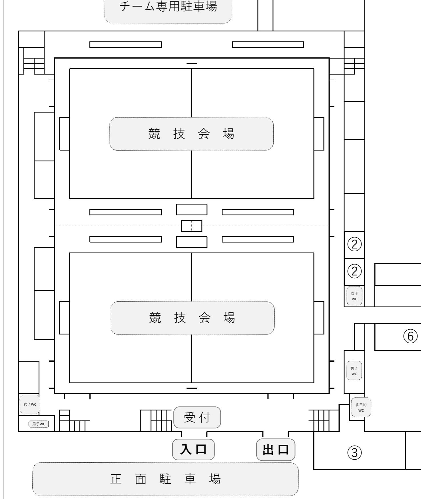
《1階平面図》
